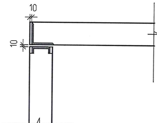
Узел 1
