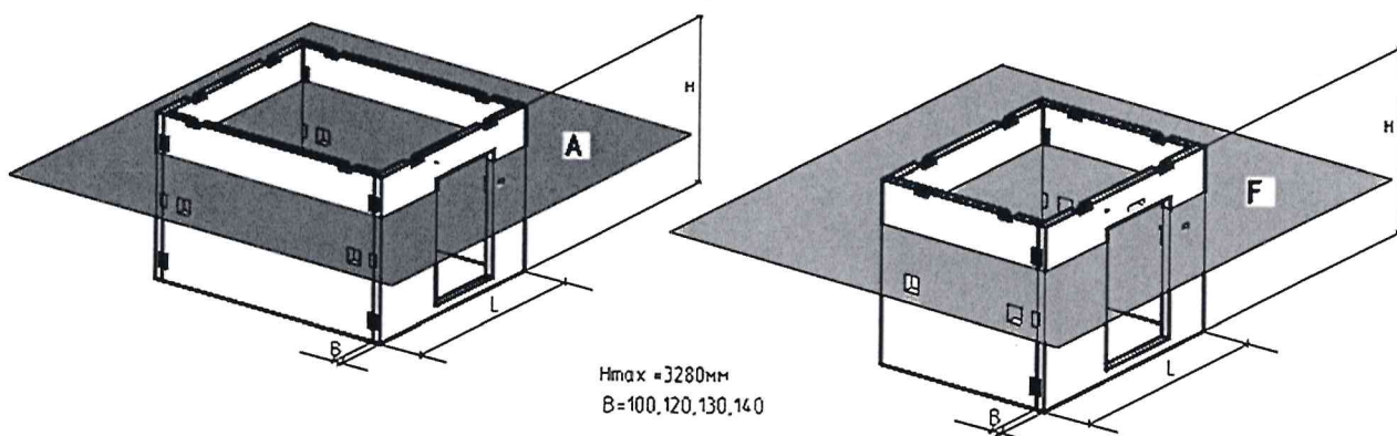
Сечение А
